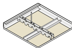
PERFILES PLADUR® PH-45 + T-45, ANGULAR Y CANAL CLIP
