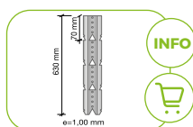
Cuelgue PF 61/T-45
