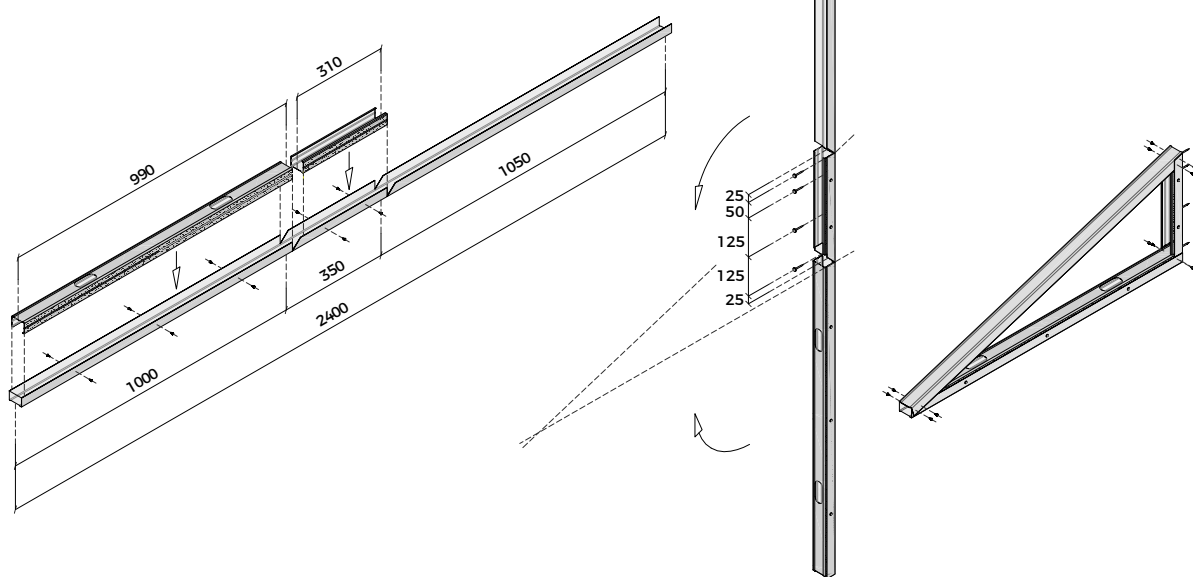
Vista isométrica
