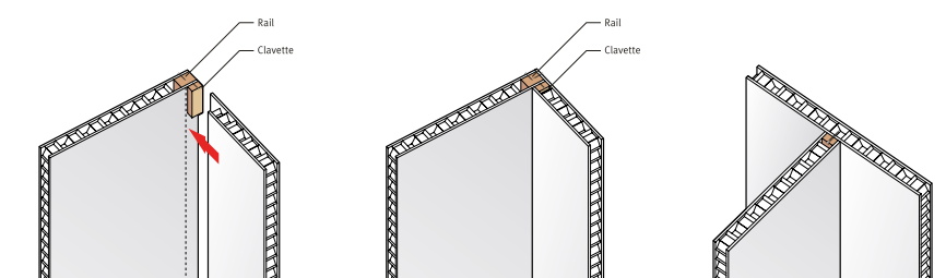
Jonction d'angle
