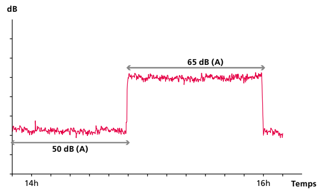
Exemple d'évolution temporelle du niveau sonore dans un local
