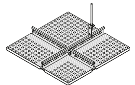
PERFILES REGISTRABLES Y ACCESORIOS PLADUR®
