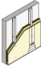
MAESTRA PLADUR ®
