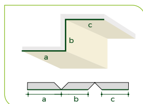
PROFORM V90 Z
