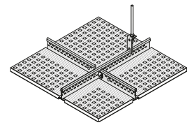
PERFIS AMOVÍVEIS E ACESSÓRIOS PLADUR ®
