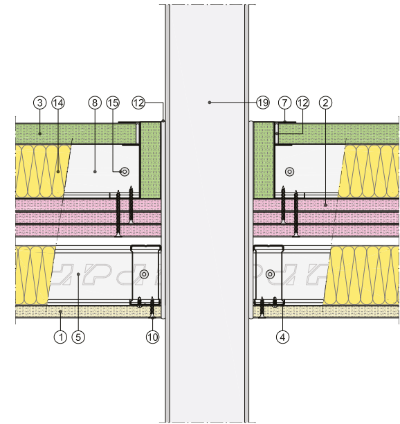
Sección horizontal
