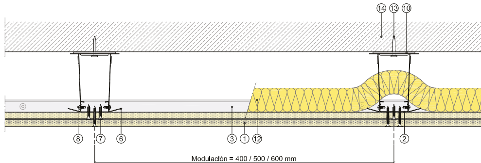
Sección vertical
