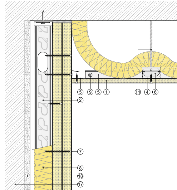
Sección vertical
