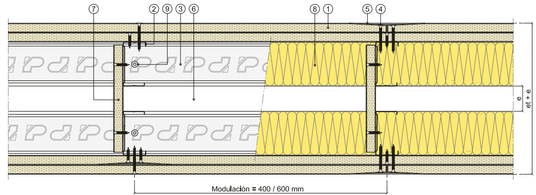
Sección horizontal
