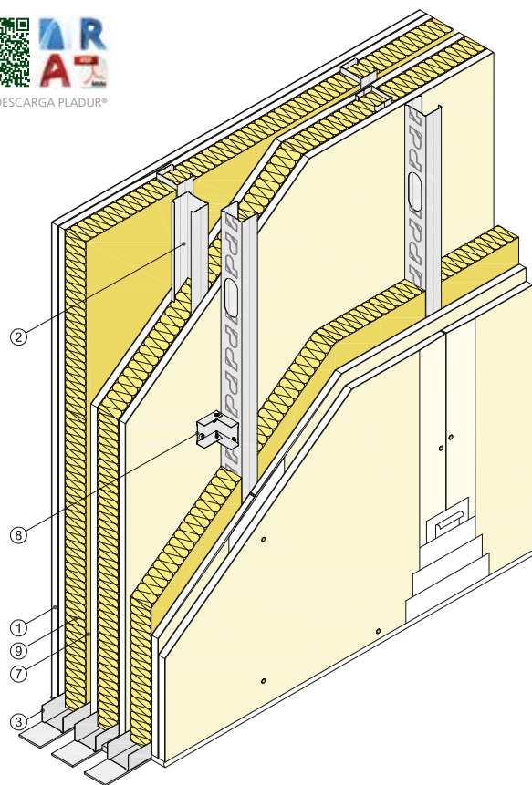
Vista isométrica
