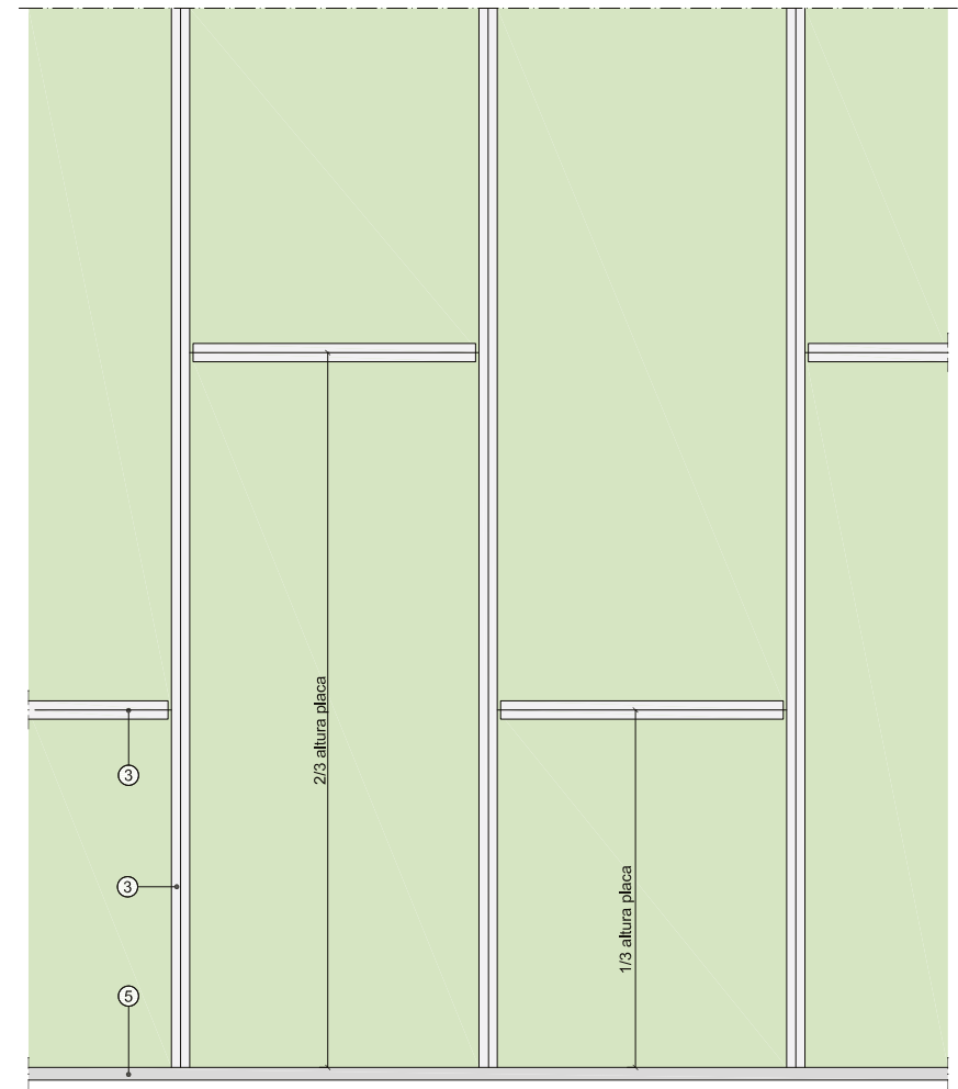
Sección vertical
