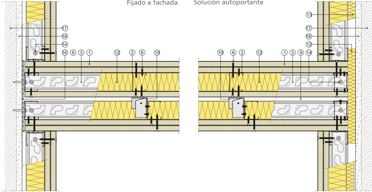
Sección horizontal
