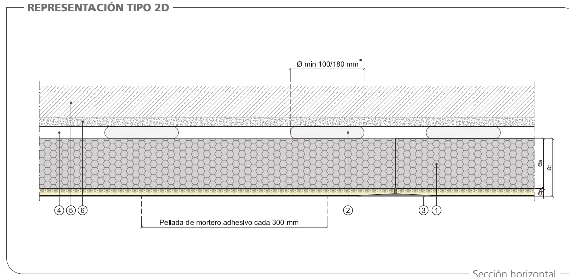
Sección horizontal
