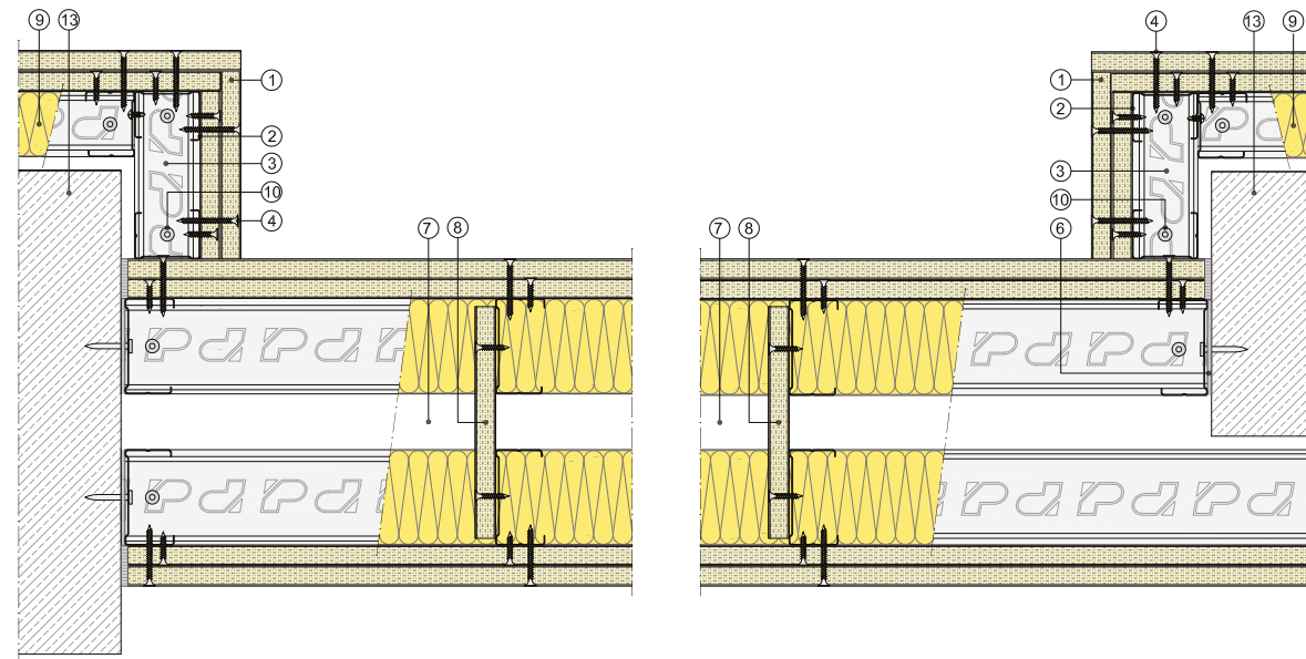
Sección horizontal
