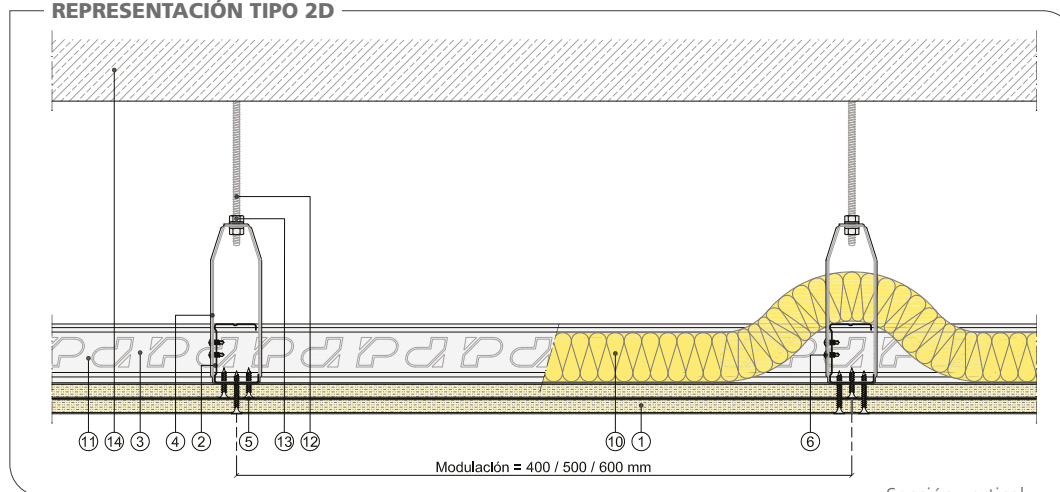
Sección vertical
