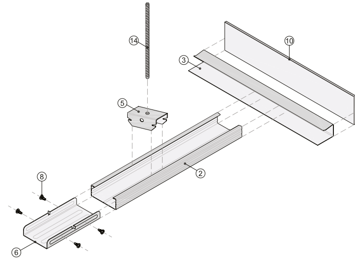
Vista isométrica
