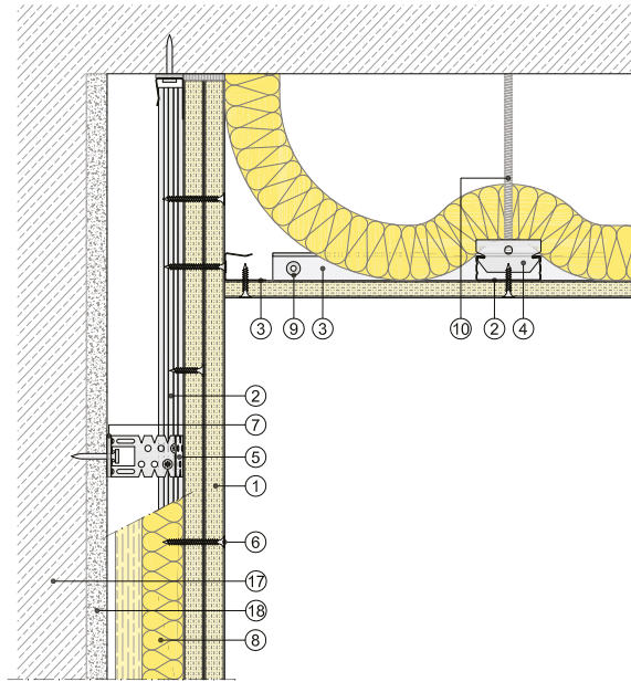
Sección vertical
