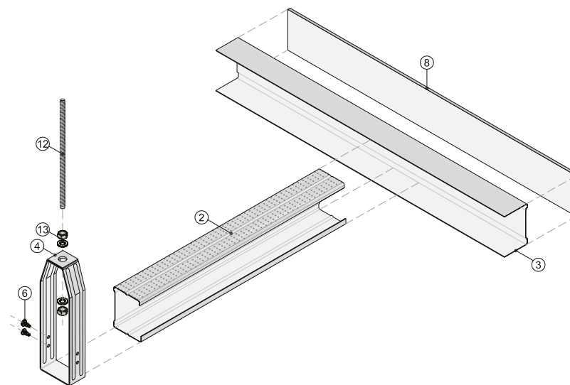
Vista isométrica
