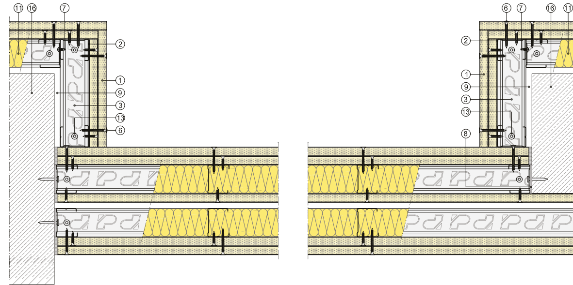
Sección horizontal
