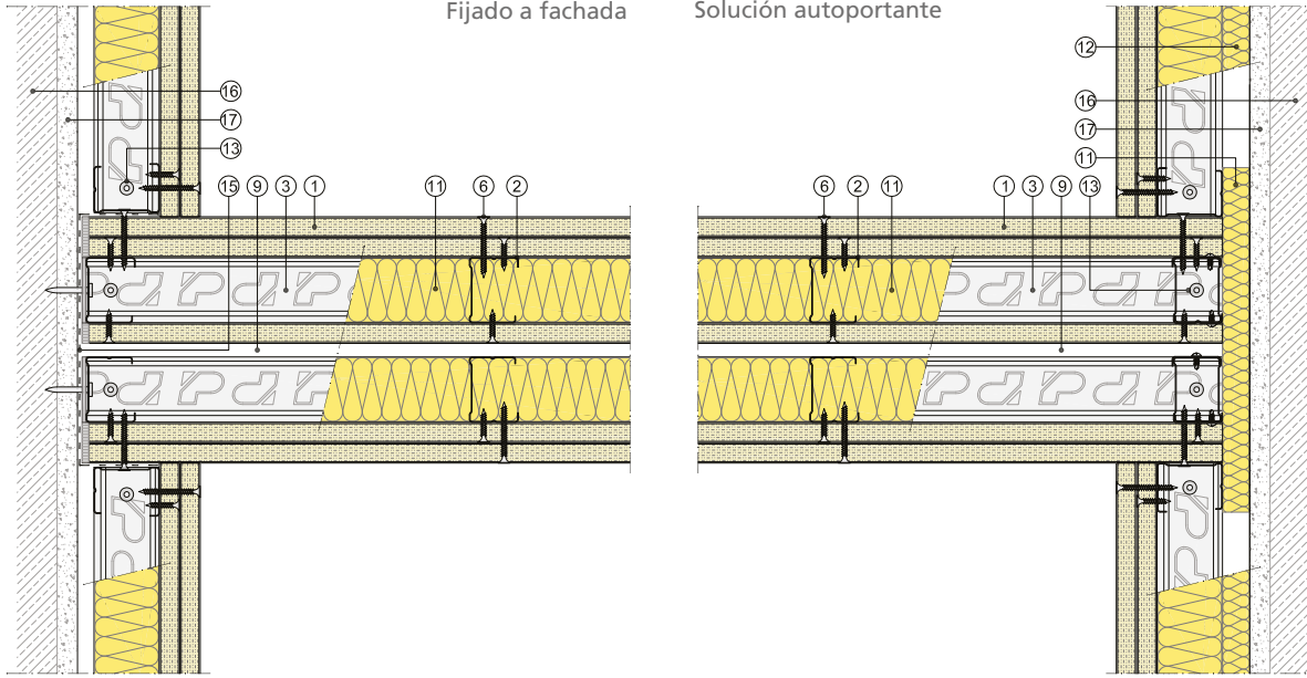
Sección horizontal
