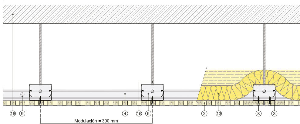
Sección vertical
