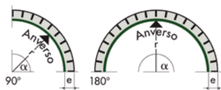
\alpha : ángulo de desarrollo e: espesor de la placa
