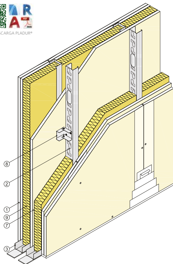
Vista isométrica
