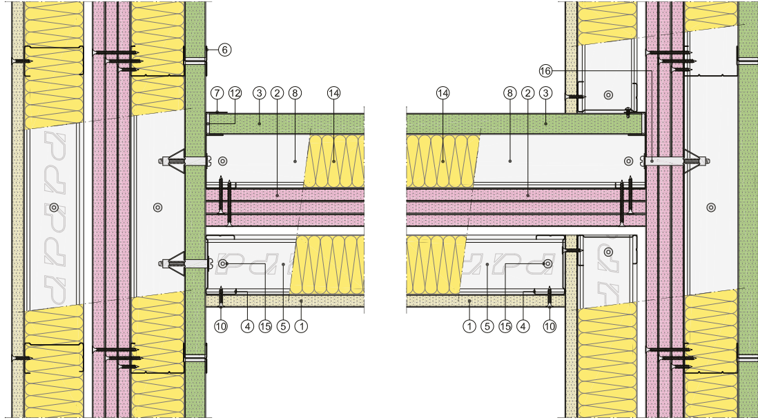
Sección horizontal
