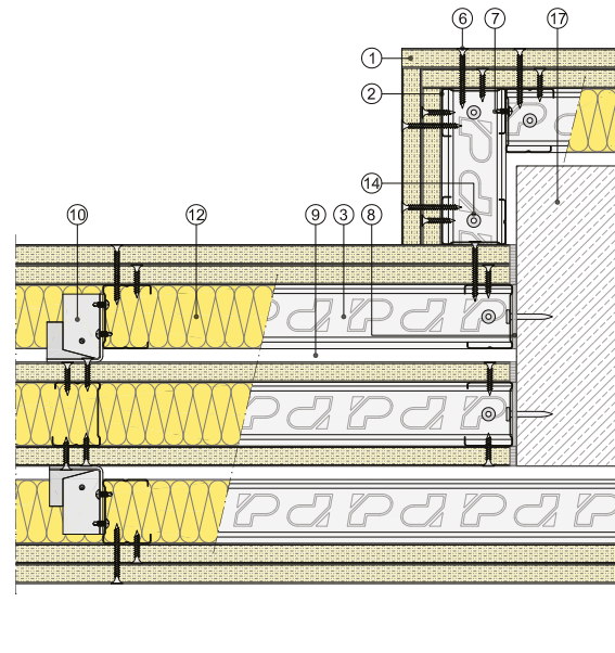
Sección horizontal
