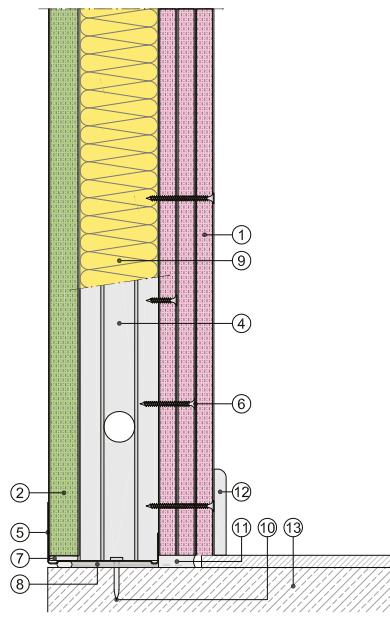
Sección vertical
