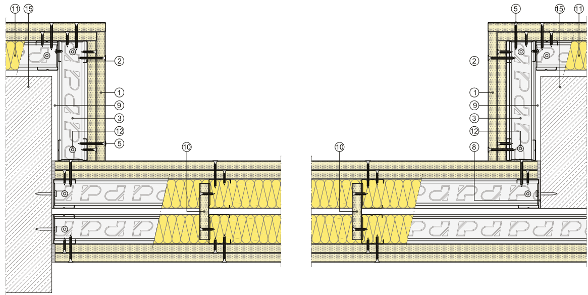
Sección horizontal
