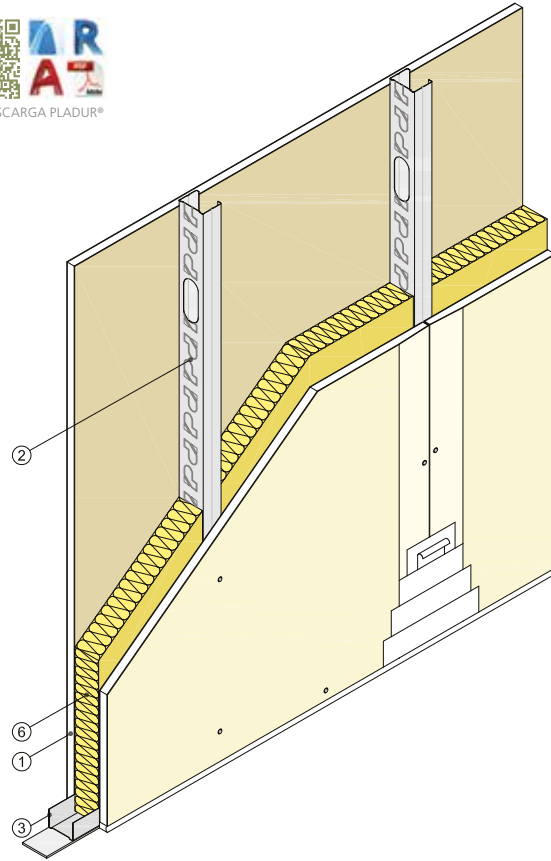
Vista isométrica
