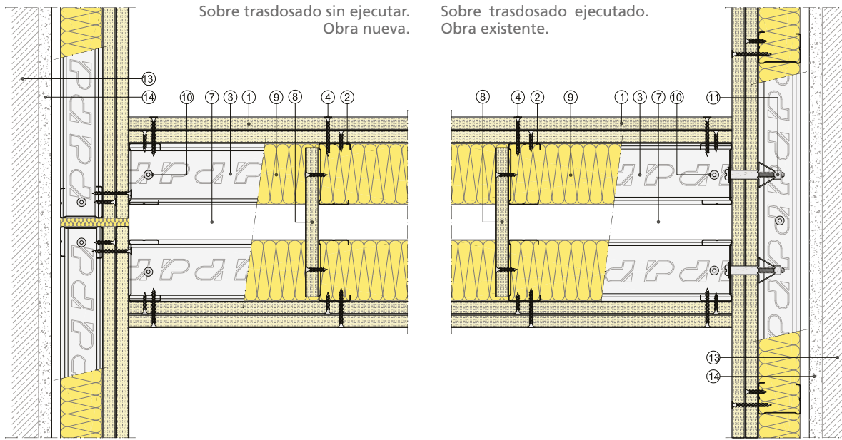
Sección horizontal
