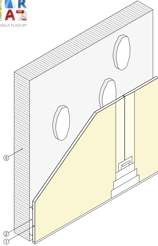
Vista isométrica
