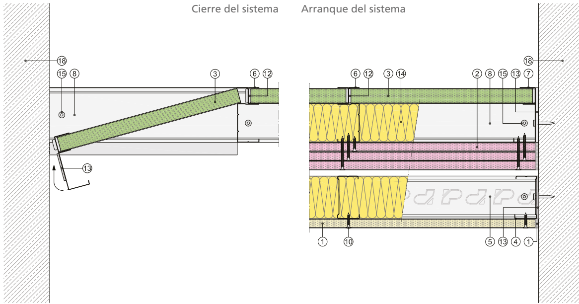
Sección horizontal
