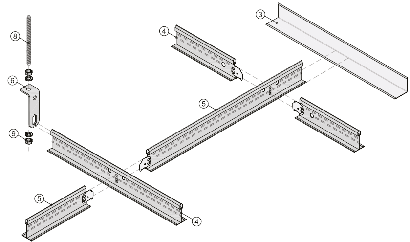
Vista isométrica
