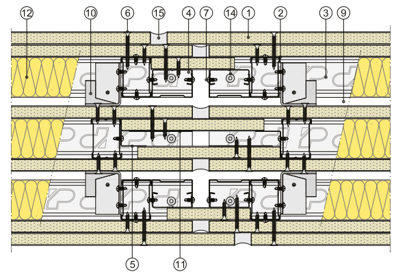
Sección horizontal
