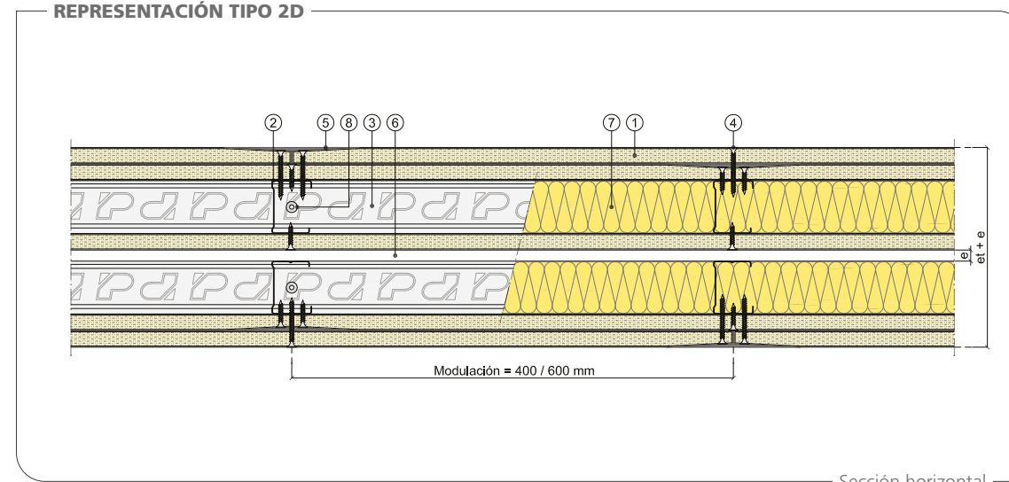
Sección horizontal
