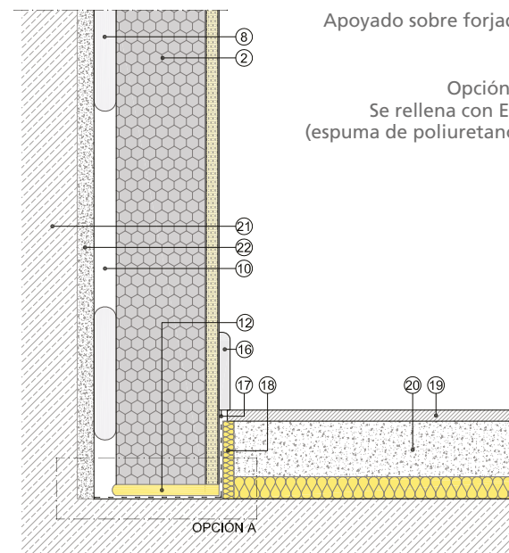
Sección vertical
