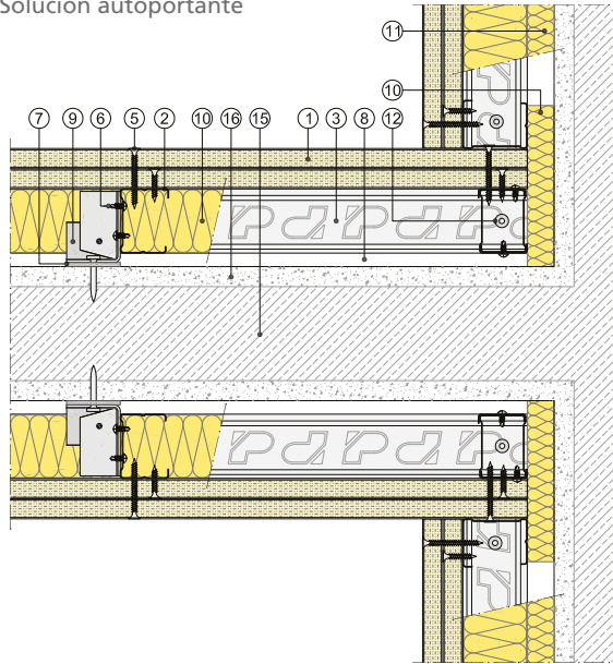
Sección horizontal
