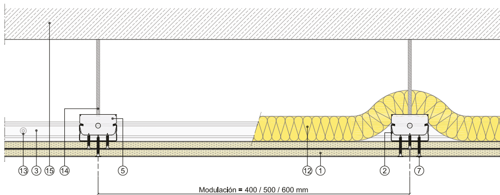
Sección vertical
