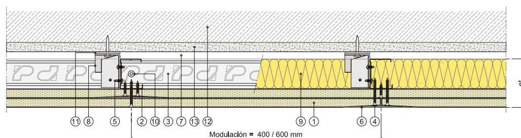
Sección horizontal
