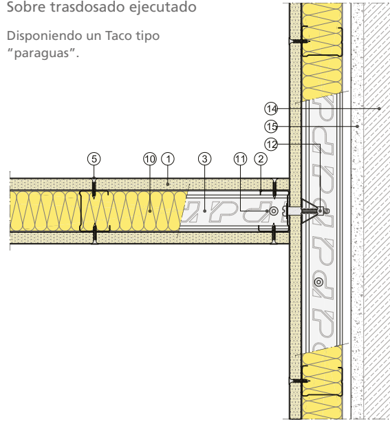
Sección horizontal
