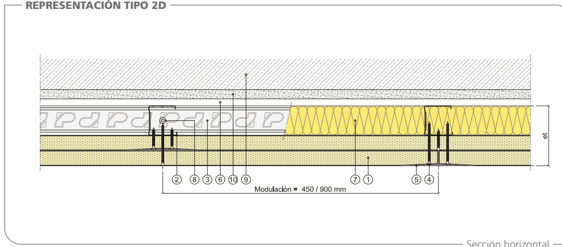
Sección horizontal
