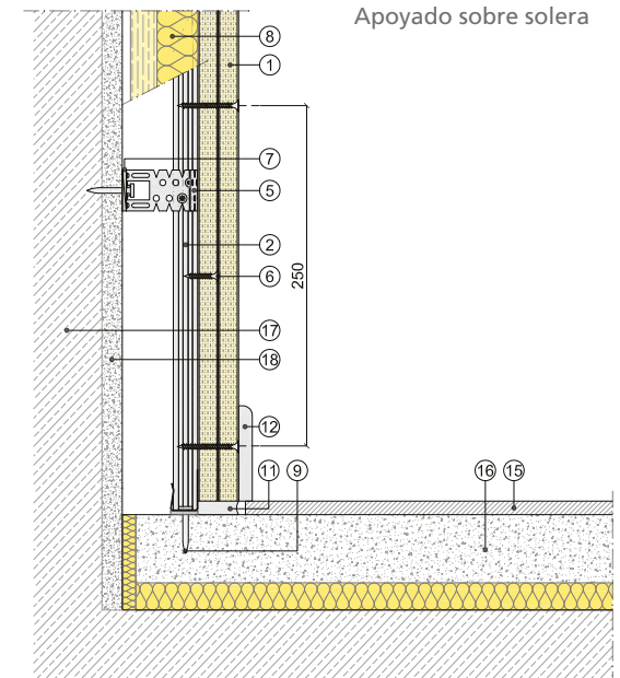
Sección vertical
