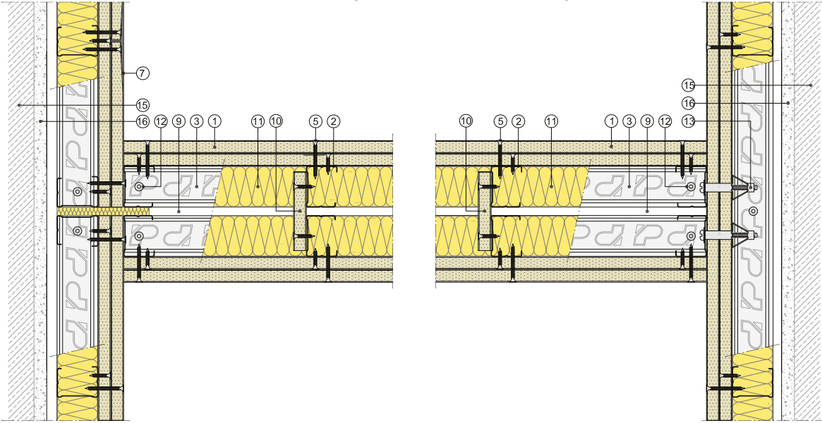
Sección horizontal
