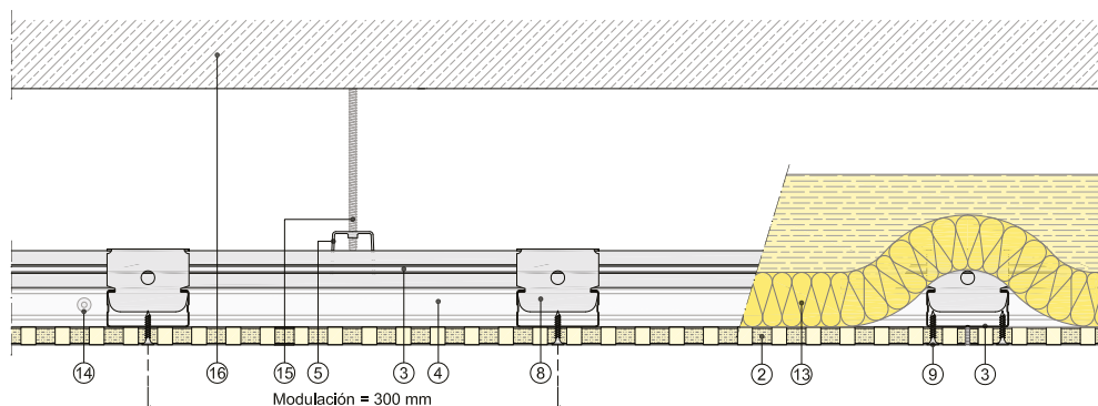
Sección vertical
