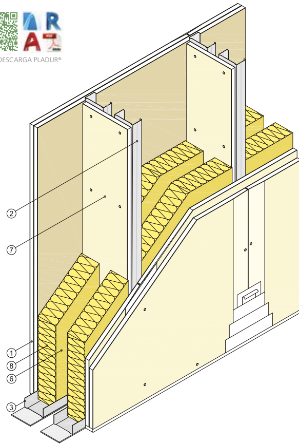
Vista isométrica
