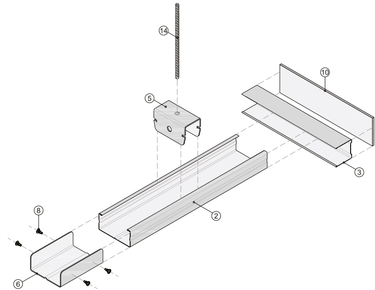
Vista isométrica
