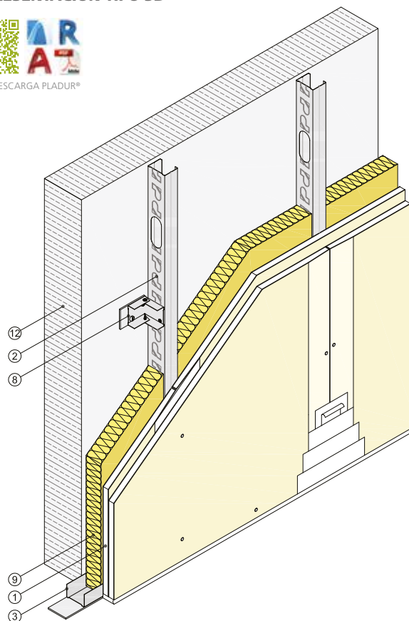
Vista isométrica
