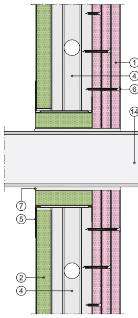
Sección vertical
