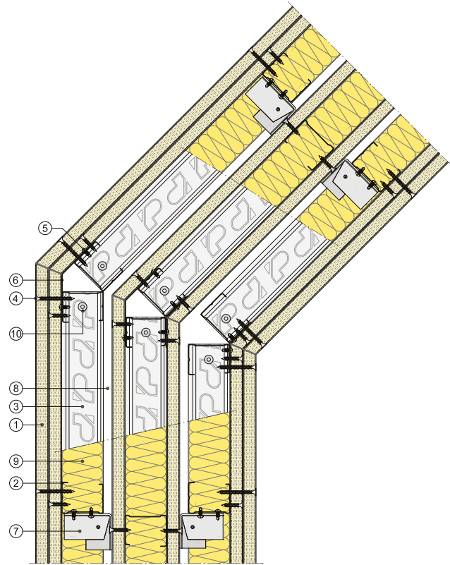
Sección horizontal
