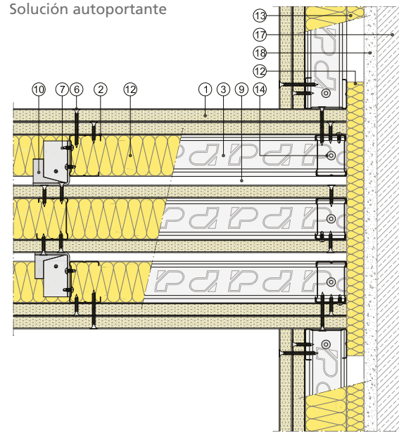
Sección horizontal
