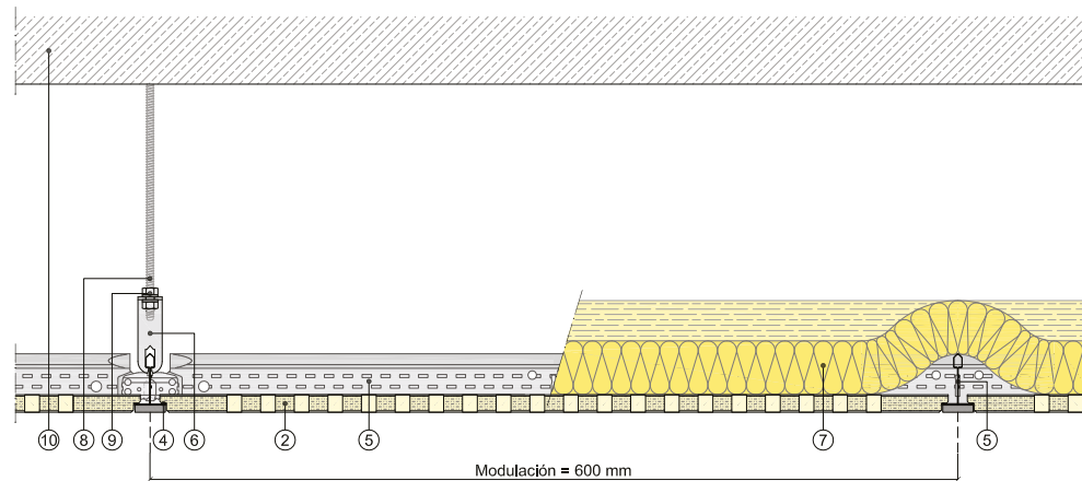
Sección vertical
