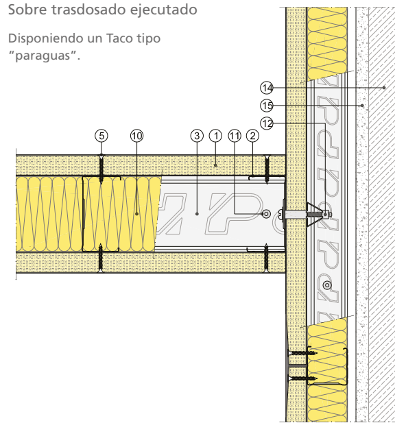
Sección horizontal
