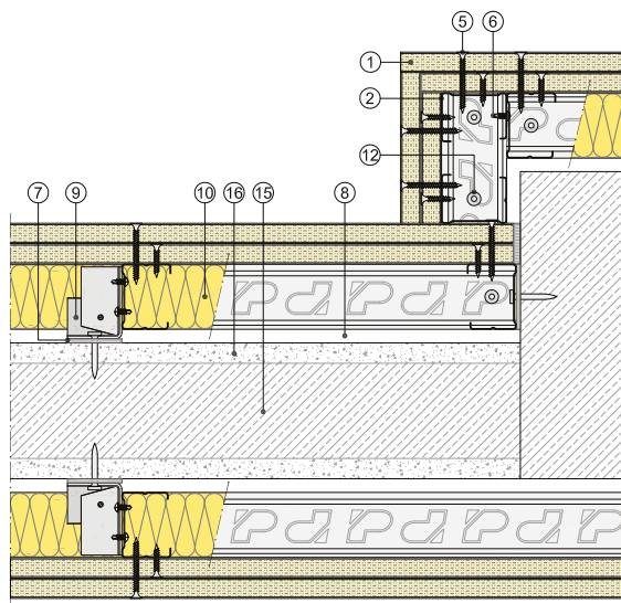
Sección horizontal
