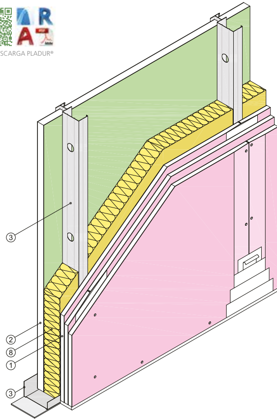
Vista isométrica
