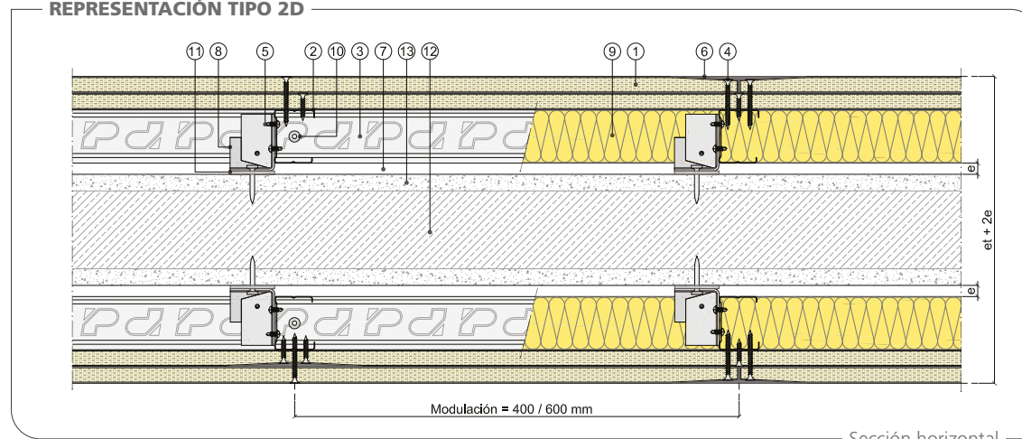
Sección horizontal
