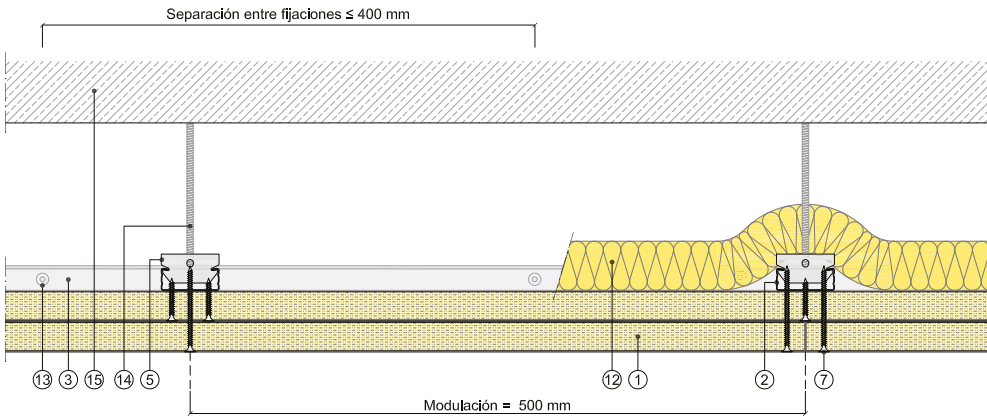
Sección vertical
