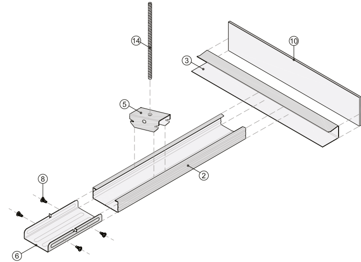
Vista isométrica
