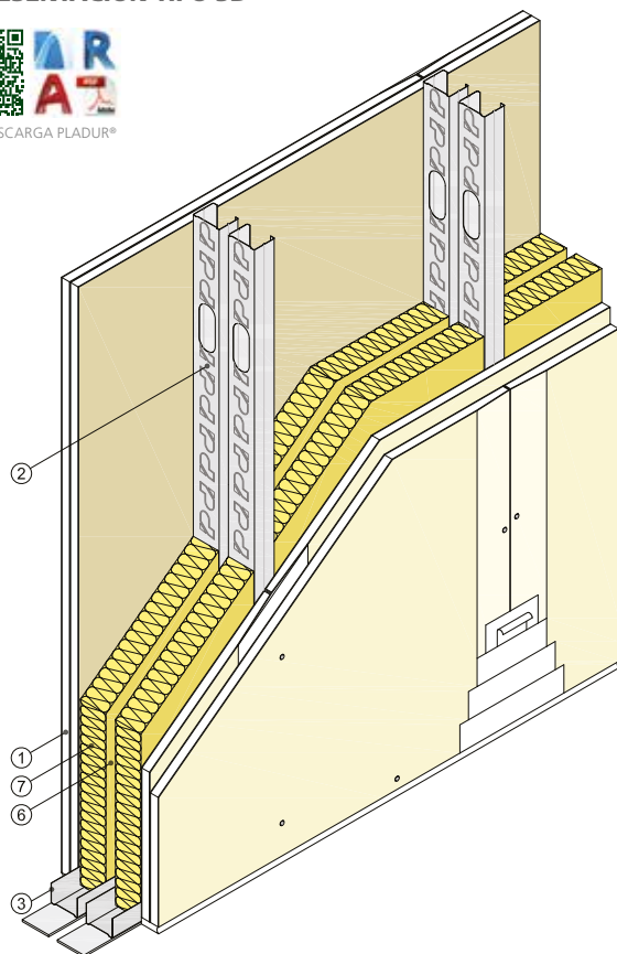
Vista isométrica
