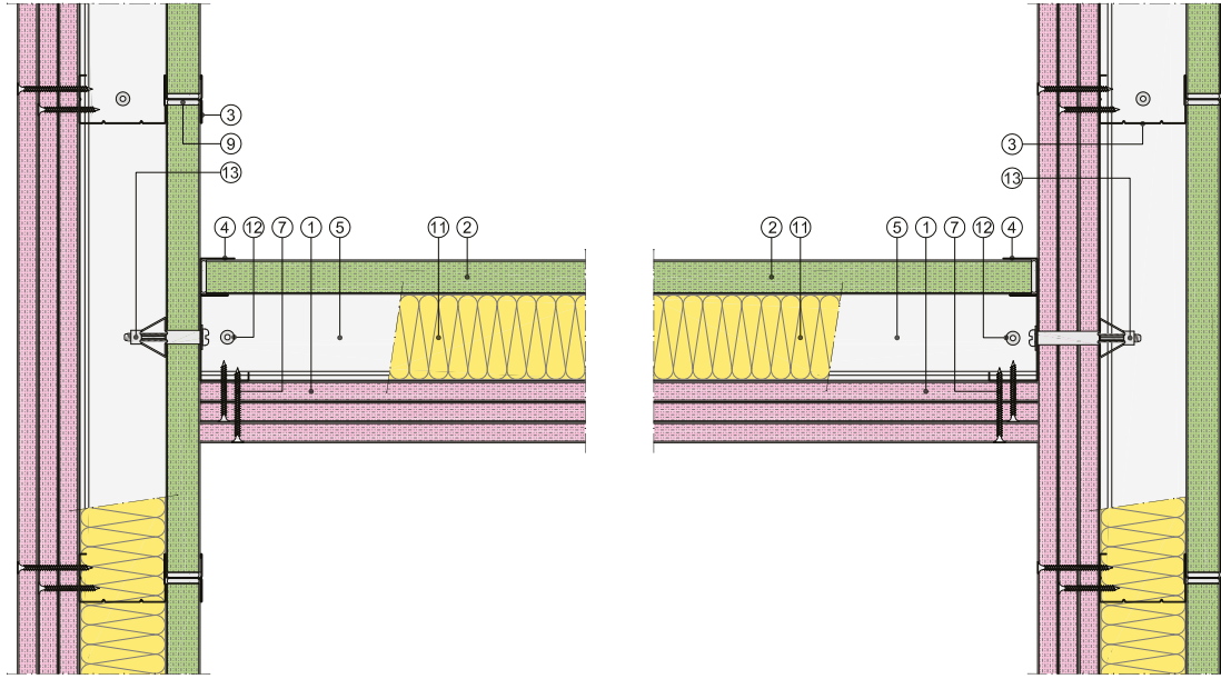
Sección horizontal
