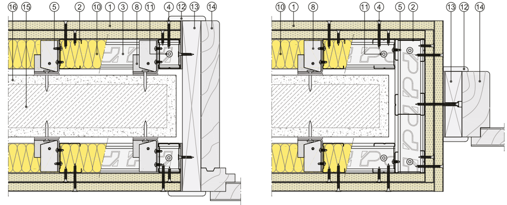
Cerco del mismo tamaño que el cerco del tabique
