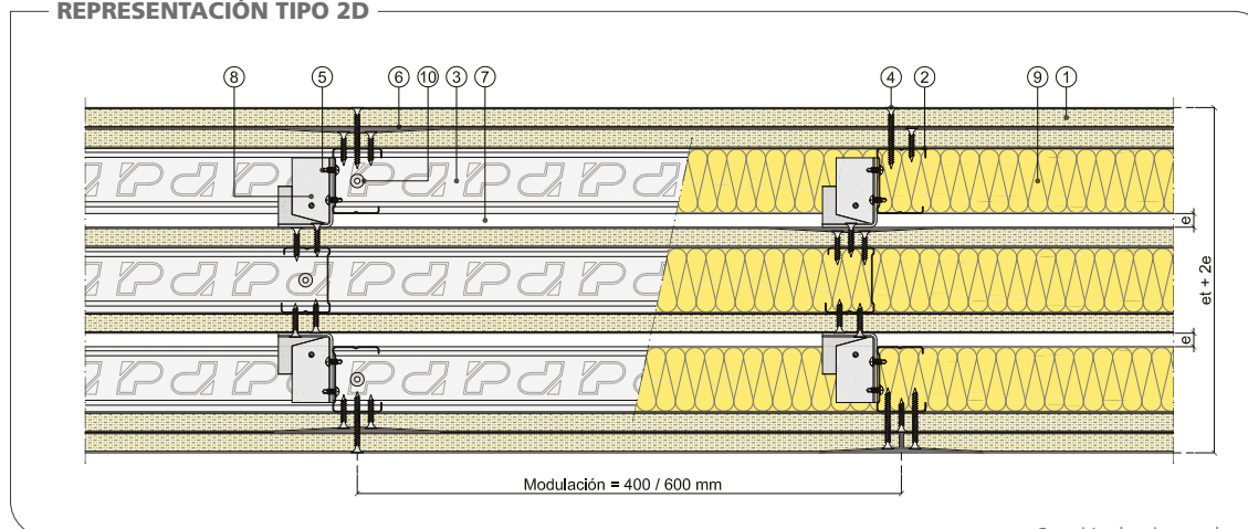
Sección horizontal
