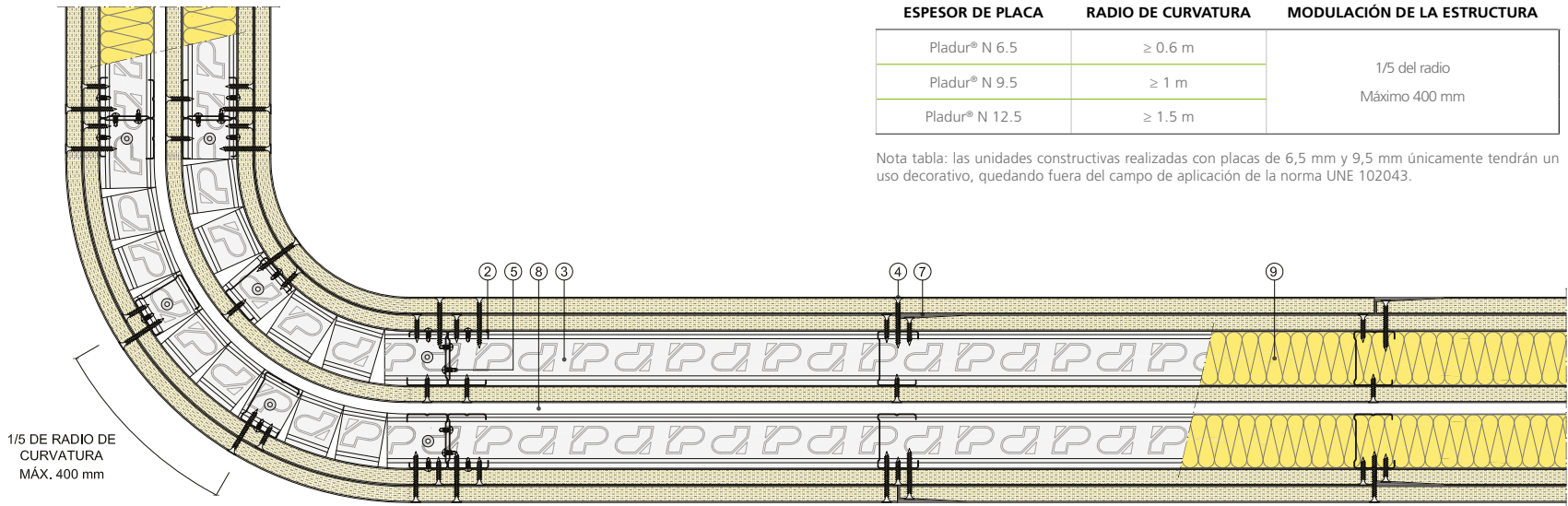
Sección horizontal
