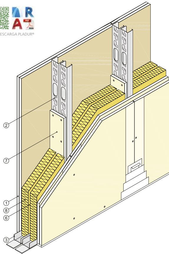
Vista isométrica
