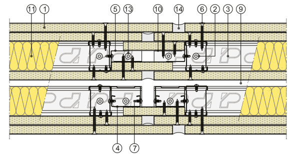
Sección horizontal
