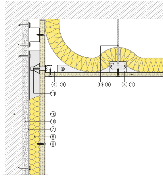
Sección vertical
