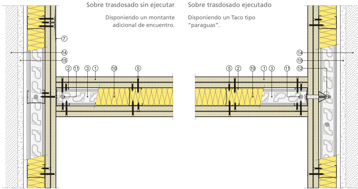
Sección horizontal
