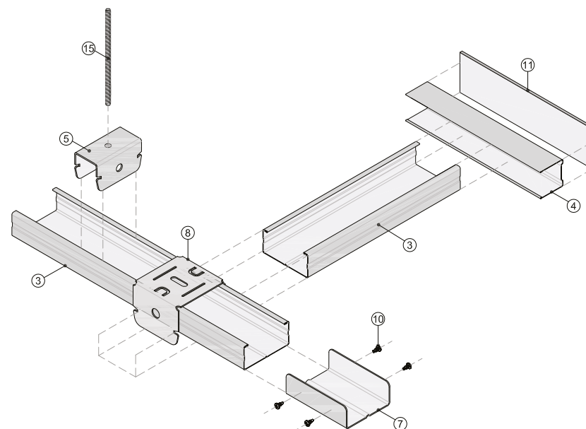
Vista isométrica
