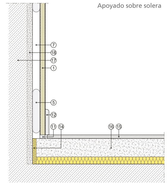
Sección vertical
