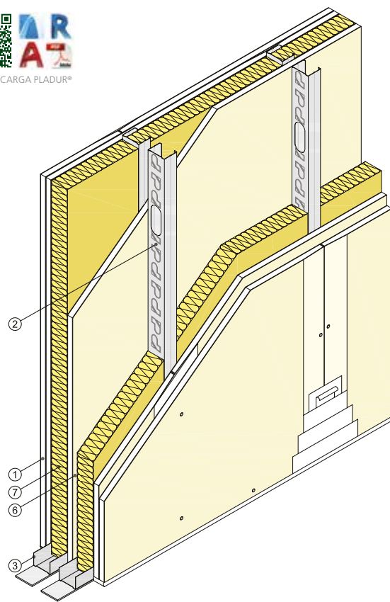
Vista isométrica
