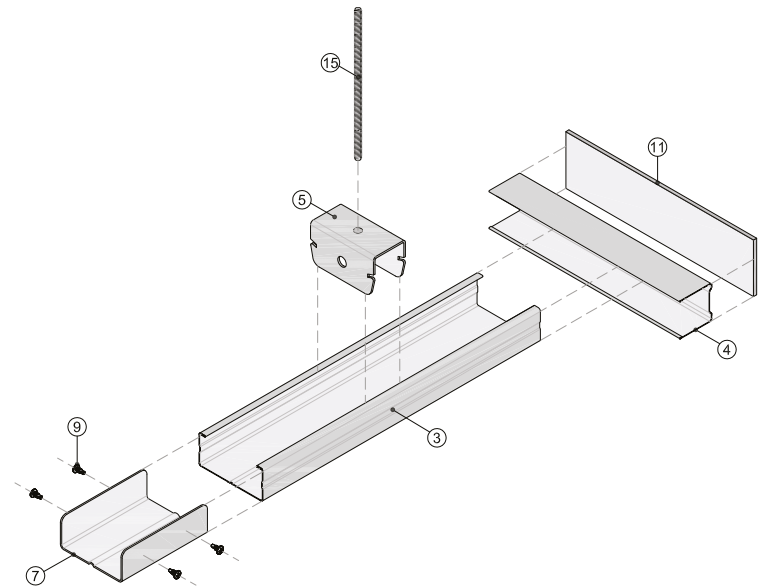
Vista isométrica
